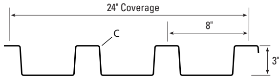
T13-A Roof
